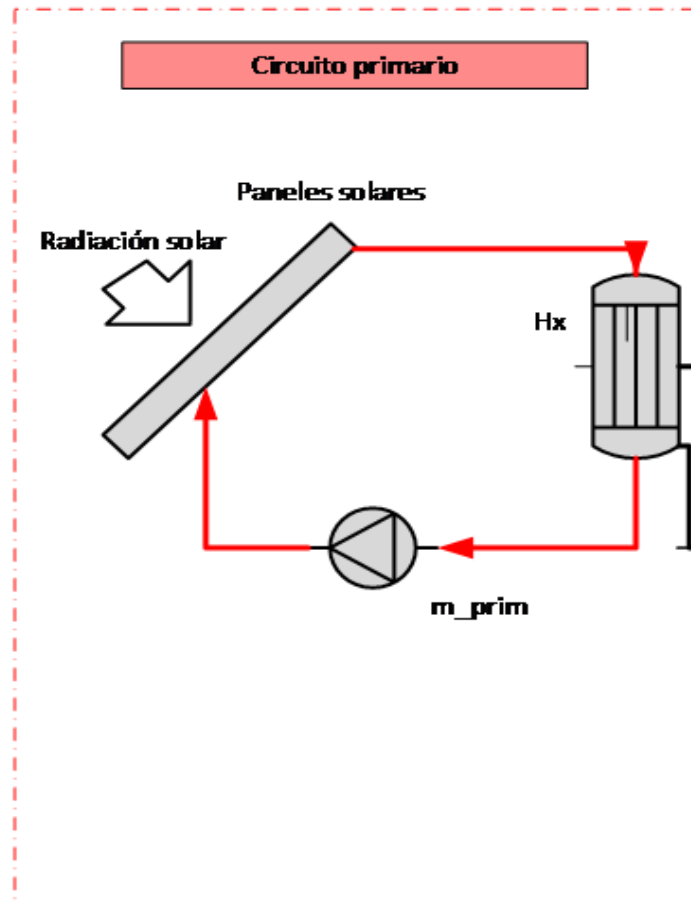
Fig. 2.3. Circuito primario de la instalación
