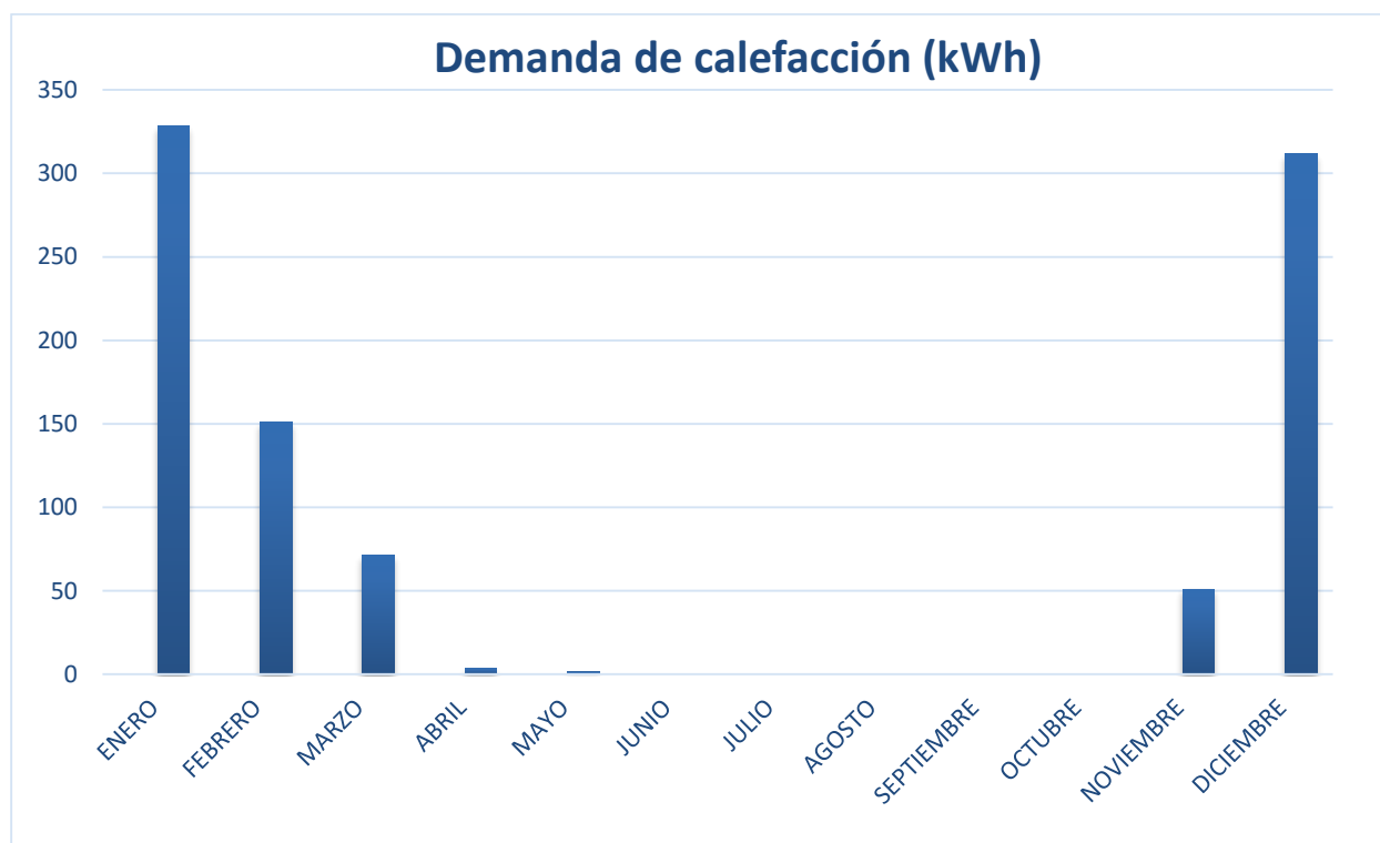
Fig. 3.11. Perfil de demanda de calefacción (KWh)
