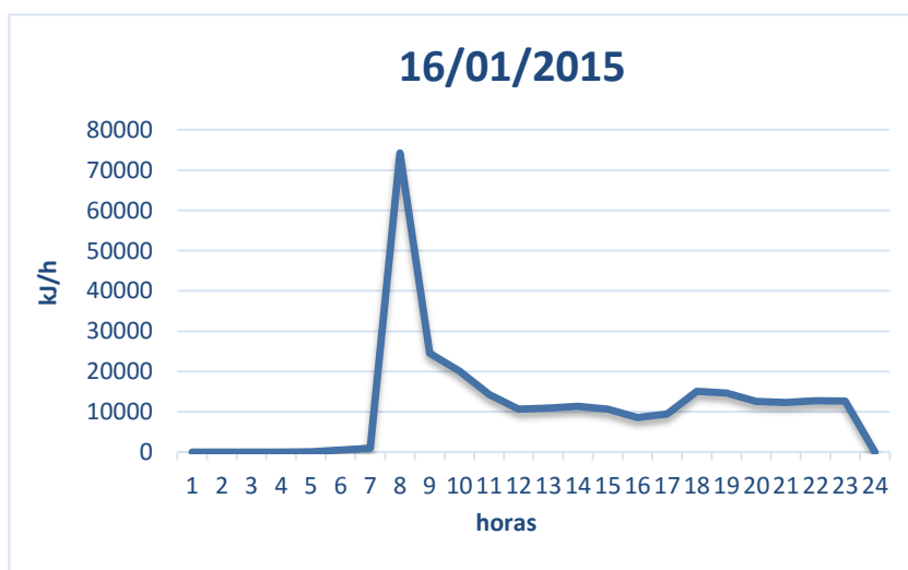
Fig. 3.12. Perfil diario de demanda de calefacción (1)
