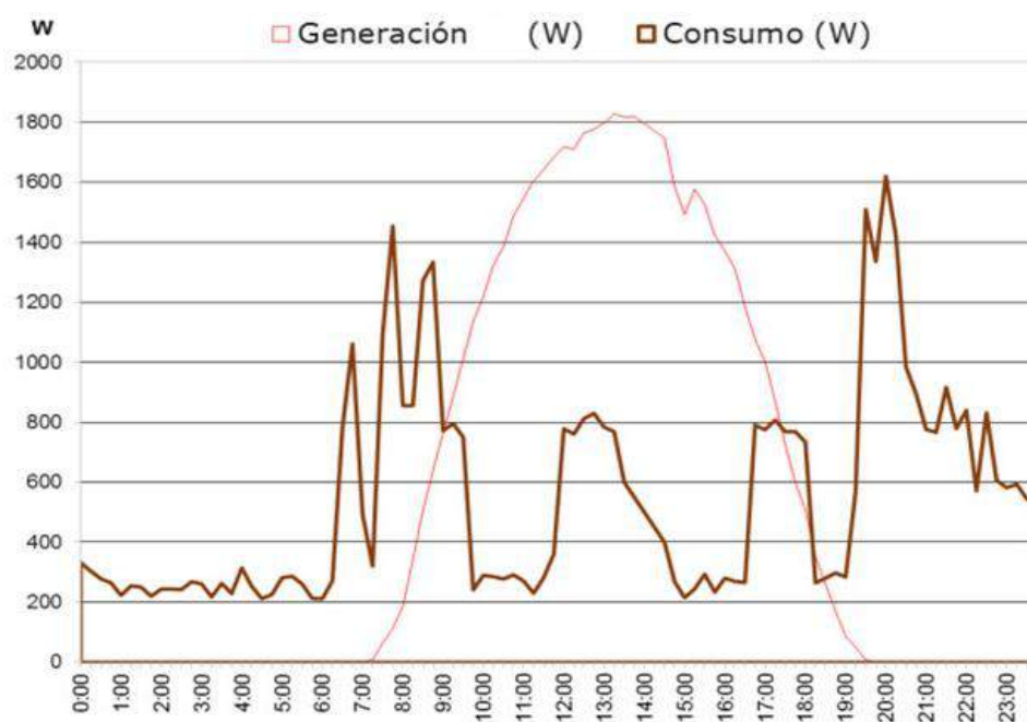
Fig. 2.10. Generación de un sistema solar térmico frente al consumo
