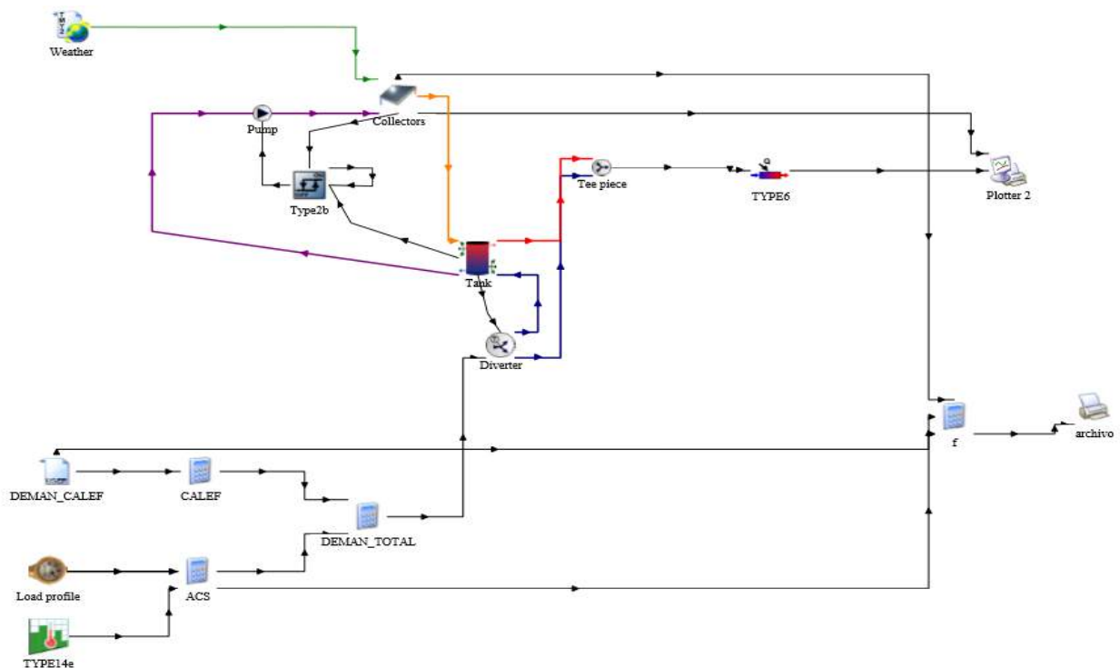
Fig. 3.1. Modelo de simulación en Trnsys
