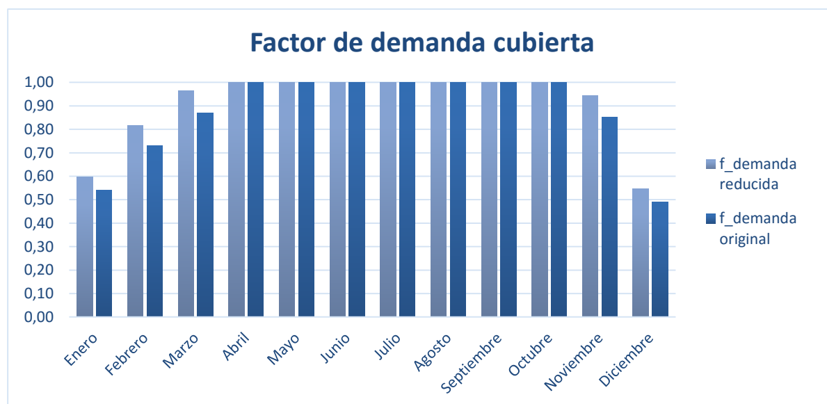
Fig. 4.3. Factor de demanda cubierta nueva VS Factor de demanda cubierta original
