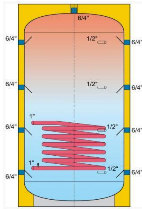
Fig. 2.11. Interior de tanque de almacenamiento de ACS
