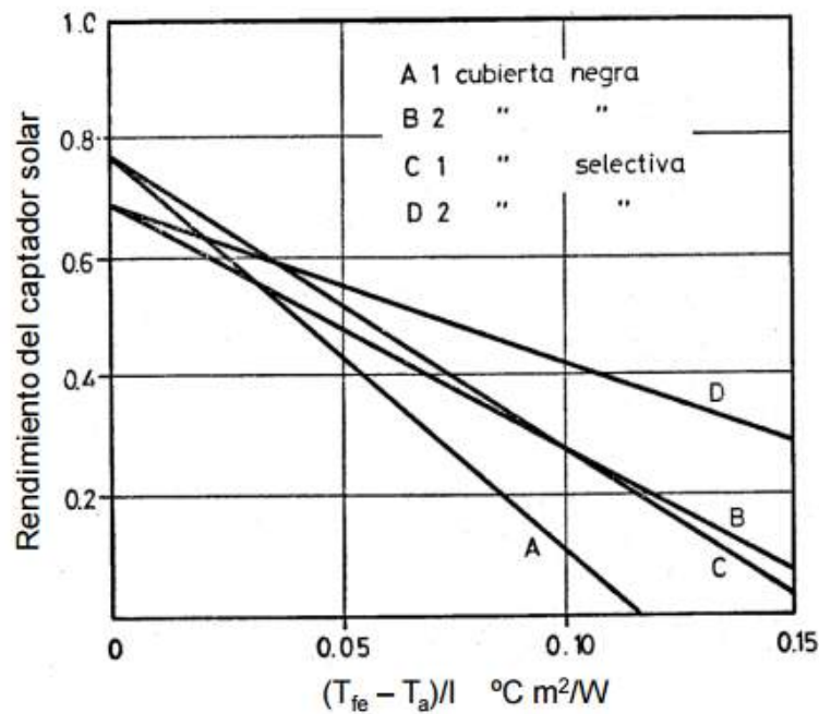
Fig. 2.7. Influencia de la temperatura de entrada del fluido y del tipo de cubierta en el rendimiento
