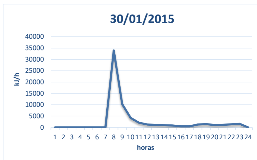
Fig. 3.13. Perfil diario de demanda de calefacción (2)
