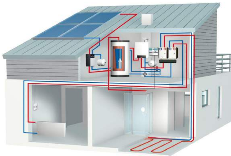
Fig. 2.1. Esquema de una vivienda con calefacción solar
