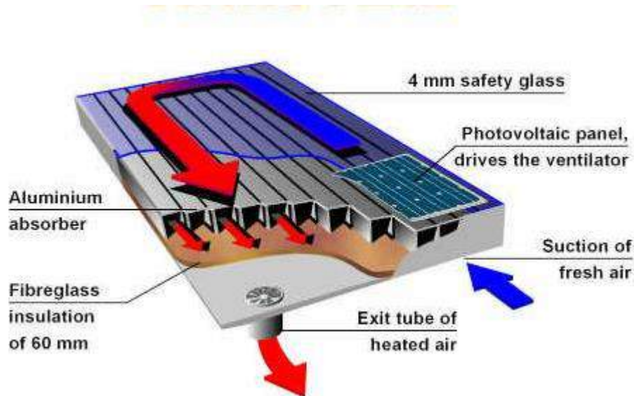
Fig. 2.8. Funcionamiento de una placa solar térmica de aire
