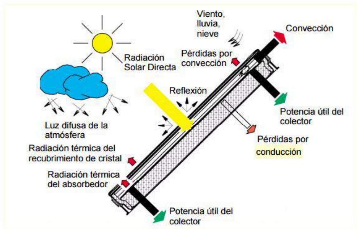
Fig. 2.6. Flujos de calor en una placa solar
