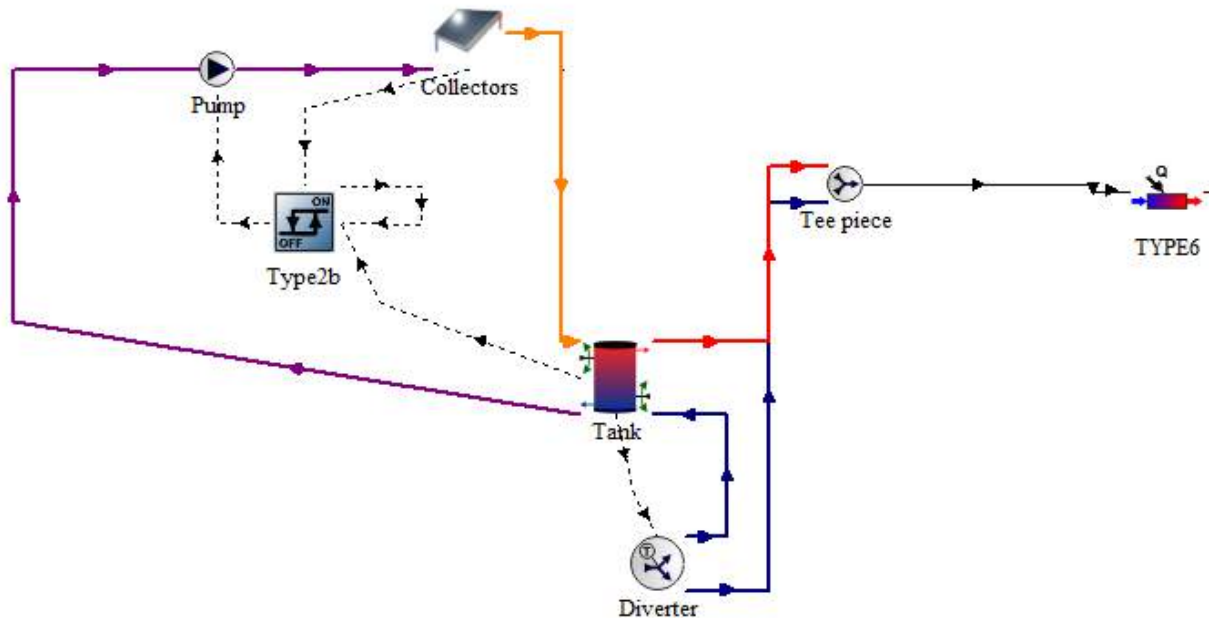
Fig. 3.2. Modelo del circuito de captación en Trnsys
