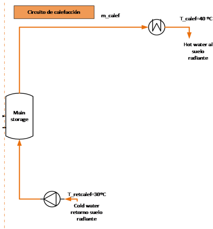
Fig. 2.5. Circuito de calefacción de la instalación
