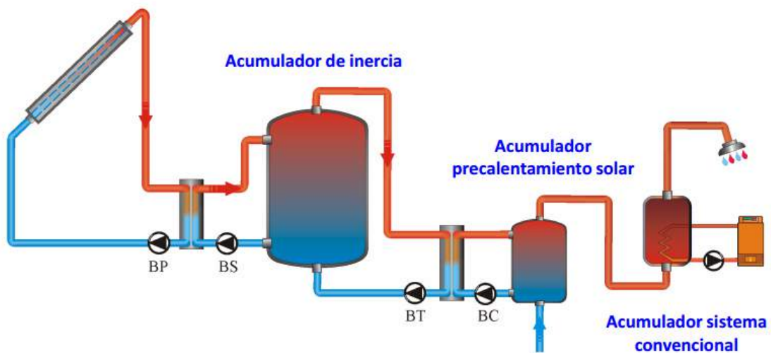
Fig. 2.12. Tipos de acumuladores en una instalación solar
