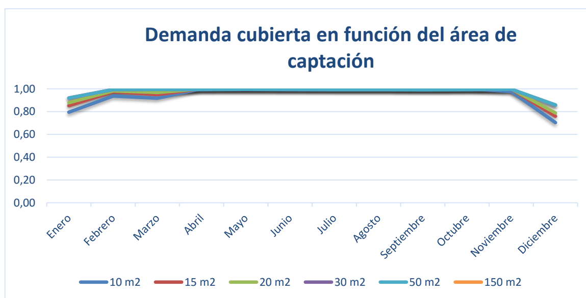
Fig. 4.1. Evolución de f en función del área de captación
