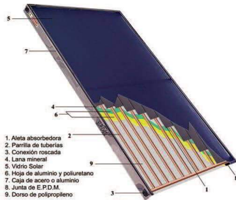
Fig 2.9. Captador solar plano de agua
