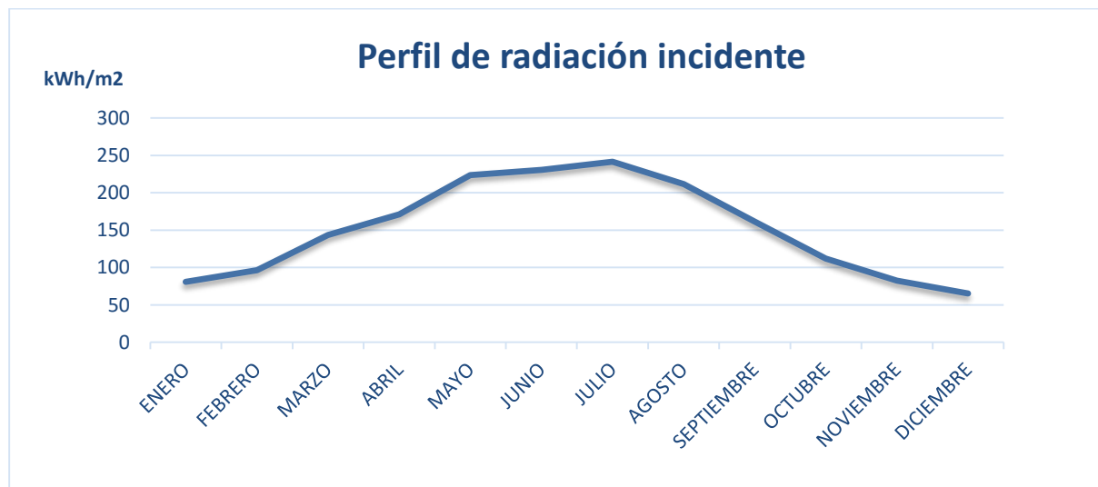
Fig. 3.22. Perfil de radiación incidente (kWh/m²)
