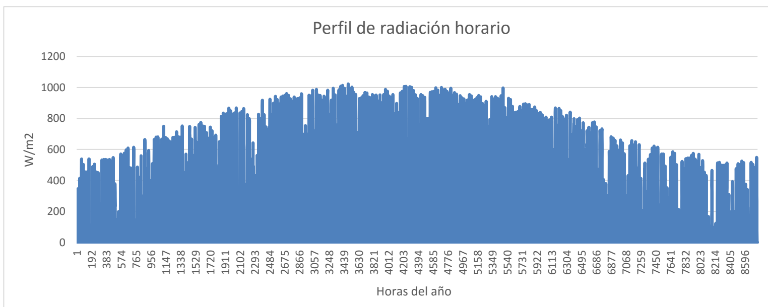
Fig. 3.4. Perfil de radiación horario en Sevilla a lo largo de un año
