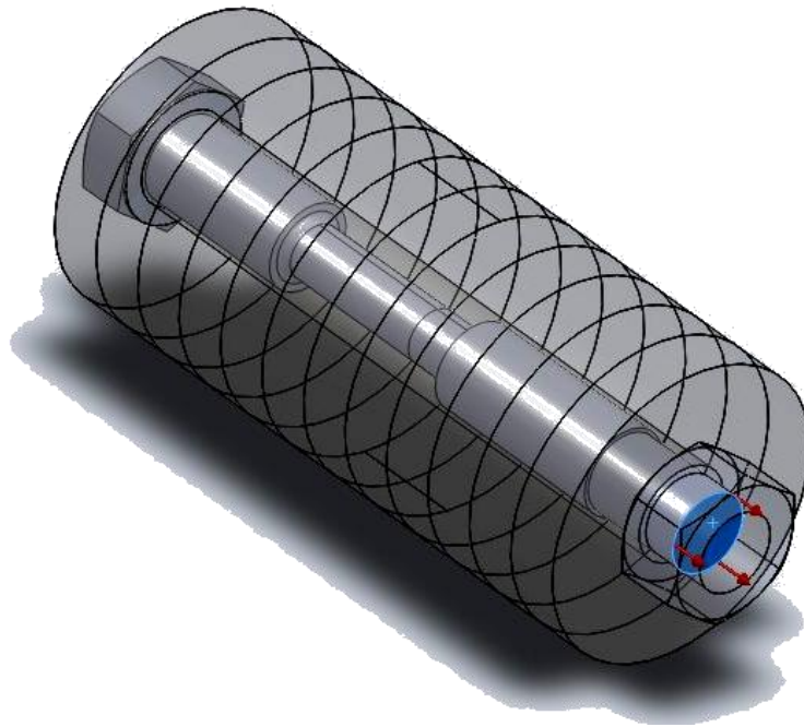
Figura 48: Modelado del apriete mediante una presión constante
