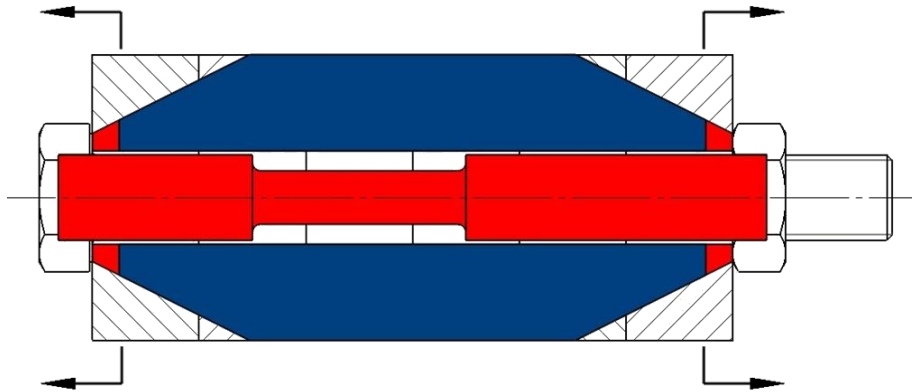
Figura 41: Actuación de la fuerza separadora en los casquillos exteriores
