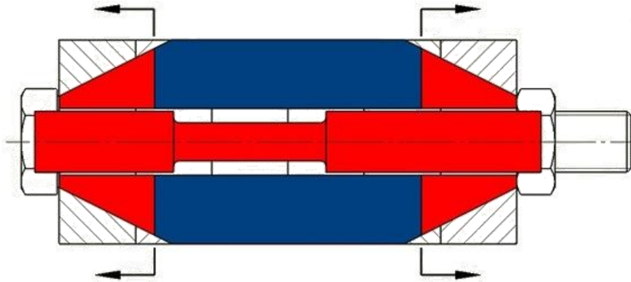
Figura 43: Actuación de la fuerza separadora en los casquillos intermedios
