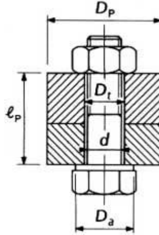
Figura 38: Parámetros necesario para el cálculo de rigidez de las piezas unidas
