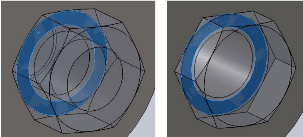
Figura 57: Caras del casquillo en contacto con la tuerca y la cabeza del tornillo
