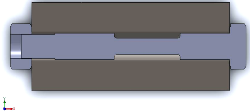
Figura 47: Sección del modelo de elementos finitos
