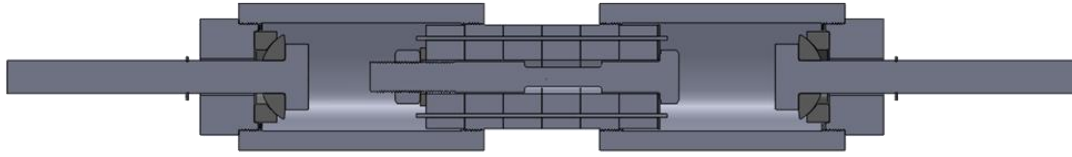
Figura 42: Montaje para aplicar la fuerza separadora desde la zona intermedia
