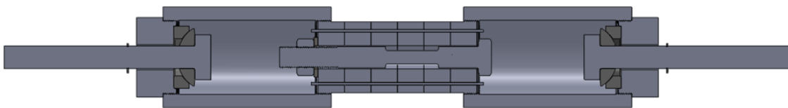
Figura 40: Montaje para aplicar la fuerza separadora desde la zona exterior
