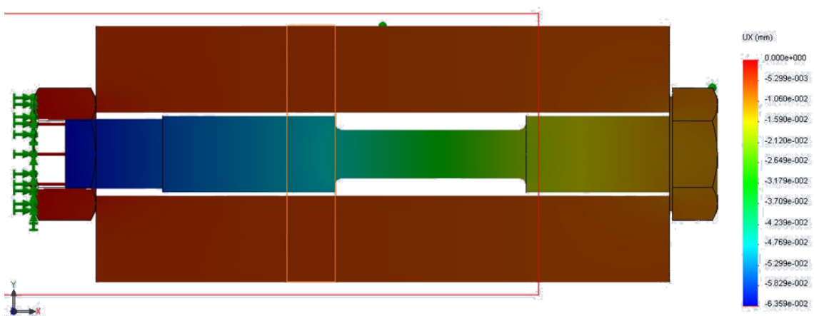
Figura 53: Desplazamientos en la dirección axial
