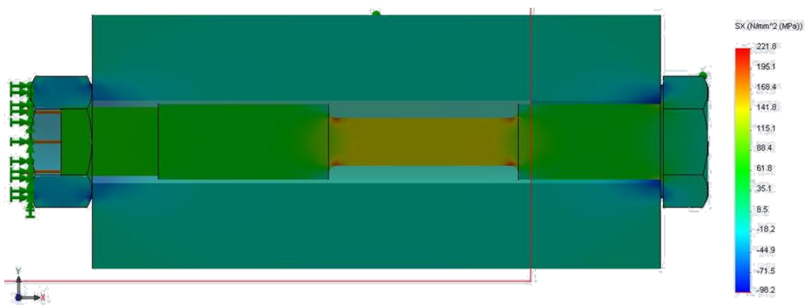
Figura 52: Tensión en la dirección axial
