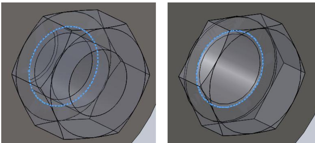
Figura 58: Aristas del casquillo en contacto con la tuerca y la cabeza del tornillo
