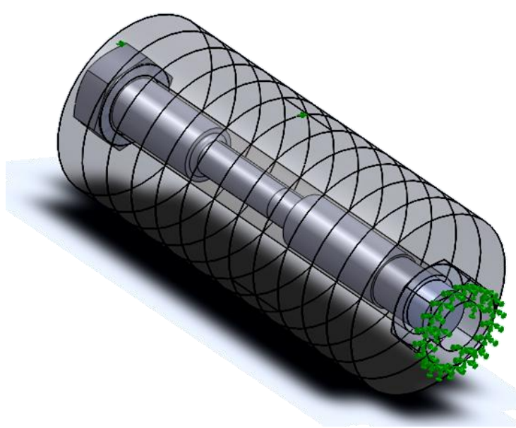
Figura 49: Condiciones de contorno del modelo de elementos finitos
