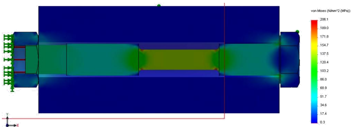
Figura 51: Tensión equivalente de Von Mises
