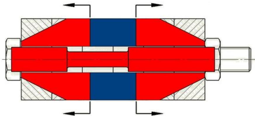
Figura 45: Actuación de la fuerza separadora en los casquillos interiores
