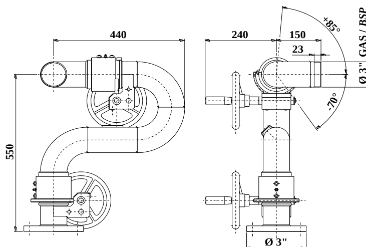
Mod. SE-KM-2V-3X 2 volantes/2 handwheel
