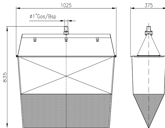
Las medidas son en mm – Dimensions are in mm
