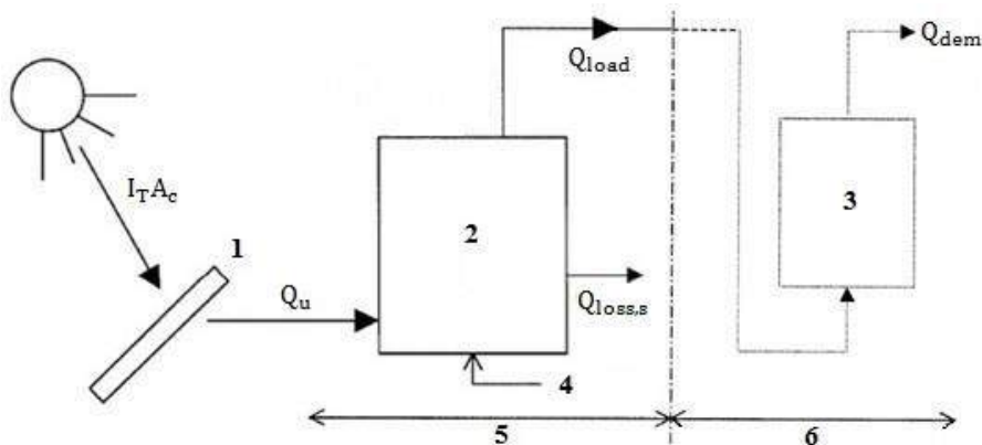
Figura 22. Sistema solar de termosifón para precalentamiento.
