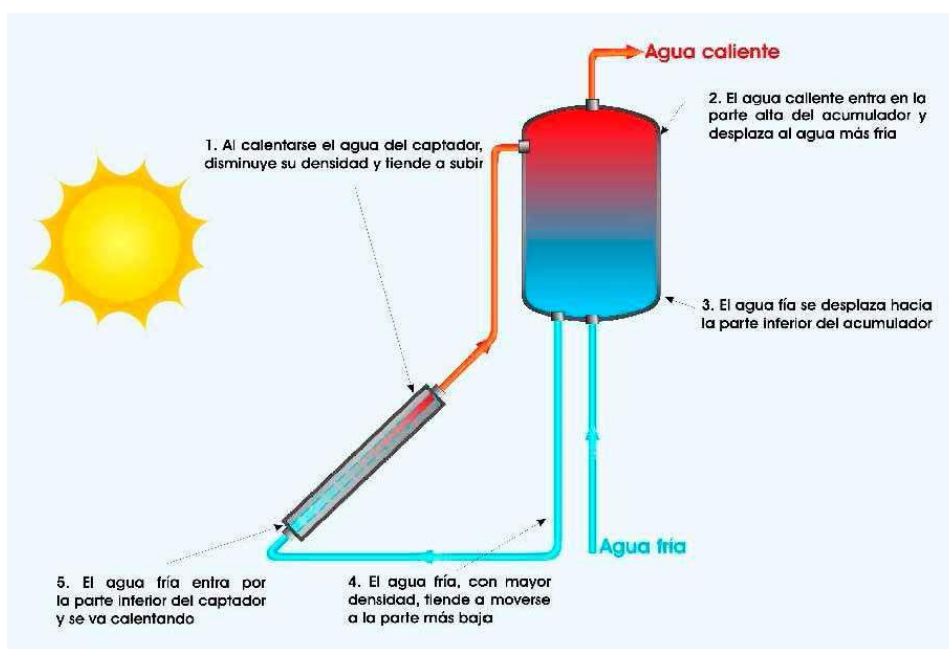
Figura 10. Sistema solar de termosifón.
