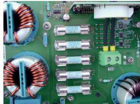
Fusibles en el inversor
