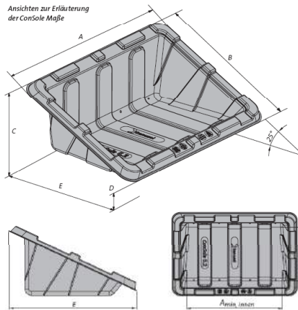
Empfohlene Maßaufnahme ConSole/PV-Modul
