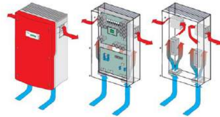
Inversor con sistema de refrigeración „OptiCool“ [imagen: SMA]
